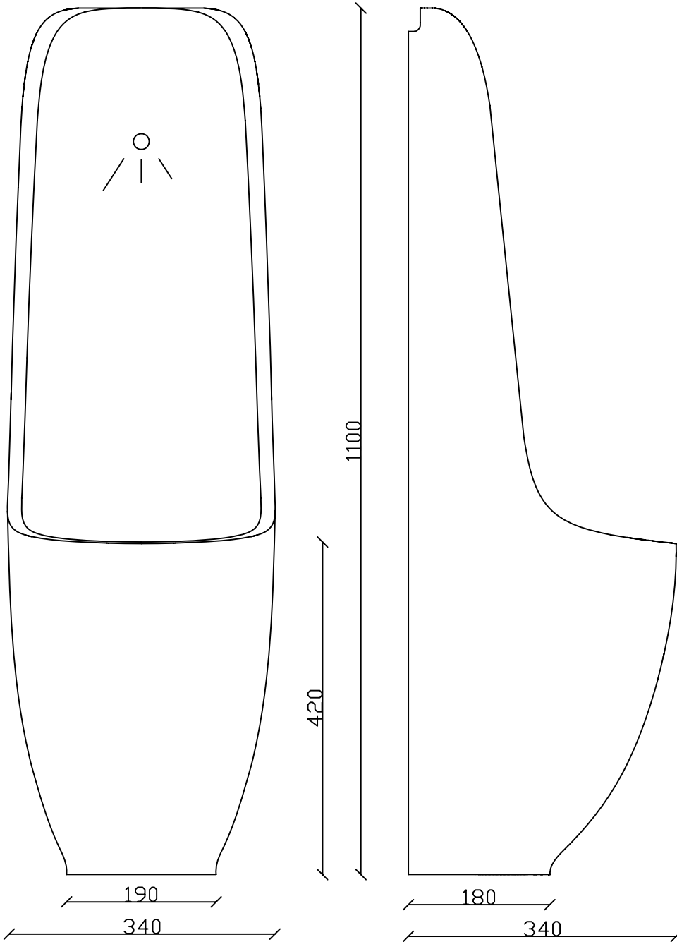
Vista frontale
