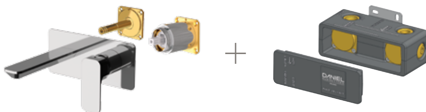
Miscelatore monocomando a incasso per lavabo, con piastra in ottone cromato, bocca lunghezza 19 cm, da abbinare al box incasso. Single-lever built-in basin mixer, with wall flange in chrome plated brass, spout length 19 cm, to match with the built-in box.
