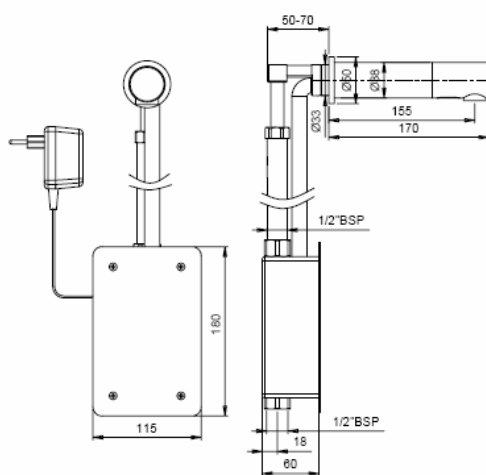
Versione a trasformatore (RUEL07E).
