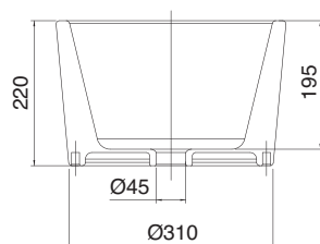
SEZIONE A-A
