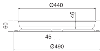
SEZIONE A-A
