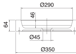
SEZIONE A-A
