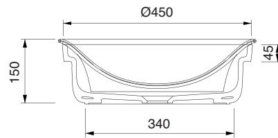
SEZIONE A-A
