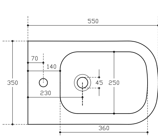
Vista dall'alto Top view Vista desde arriba Vue de haut
