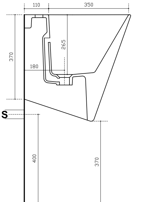
Sezione A-A Section A-A Sección A-A Section A-A
