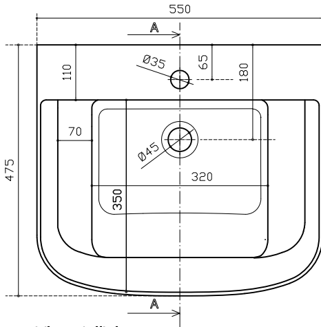
Vista dall'alto Top view Vista desde arriba Vue du haut
