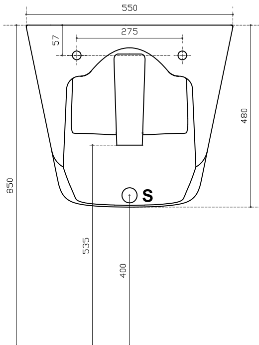
Vista posteriore Rear View Vista posterior Vue en arrière
