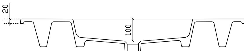
Sezione A-A
