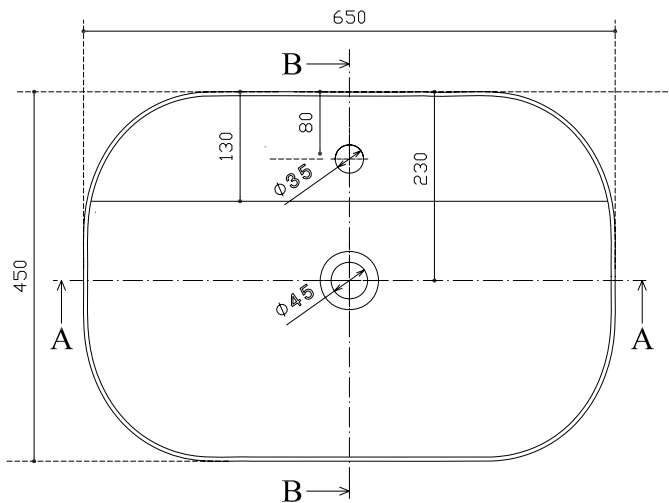
Vista dall'alto View from above Vista desde arriba Vue de dessus
