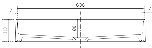
Sezione A-A Section A-A Sección A-A Section A-A
