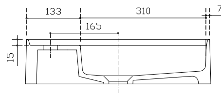
Sezione B-B Section B-B Sección B-B Section B-B
