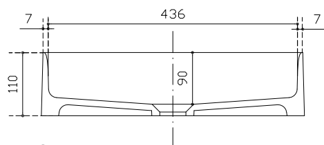
Sezione A-A Section A-A Sección A-A Section A-A
