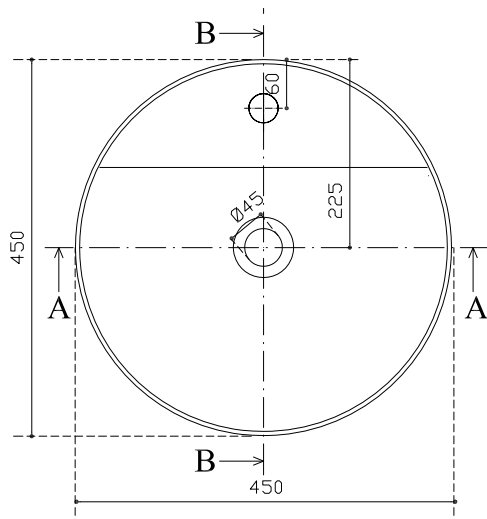
Vista dall'alto View from above Vista desde arriba Vue de dessus
