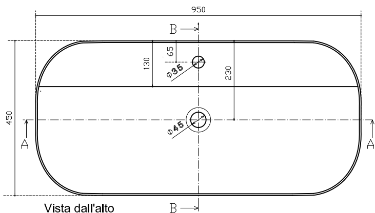
Vista dall'alto View from above Vista desde arriba Vue du haut
