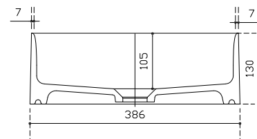
Sezione B-B Section B-B Sección B-B Section B-B
