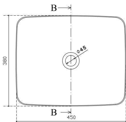
Vista dall'alto View from above Vista desde arriba Vue de dessus
