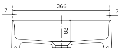
Sezione B-B Section B-B Sección B-B Section B-B
