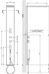
SEZIONE A-A
