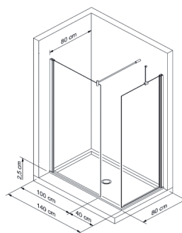
Combinazione C Combination C
