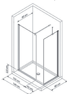
Combinazione B Combination B
