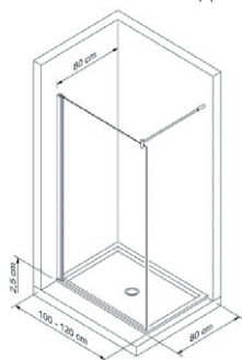
Combinazione A Combination A
