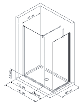
Combinazione D Combination D
