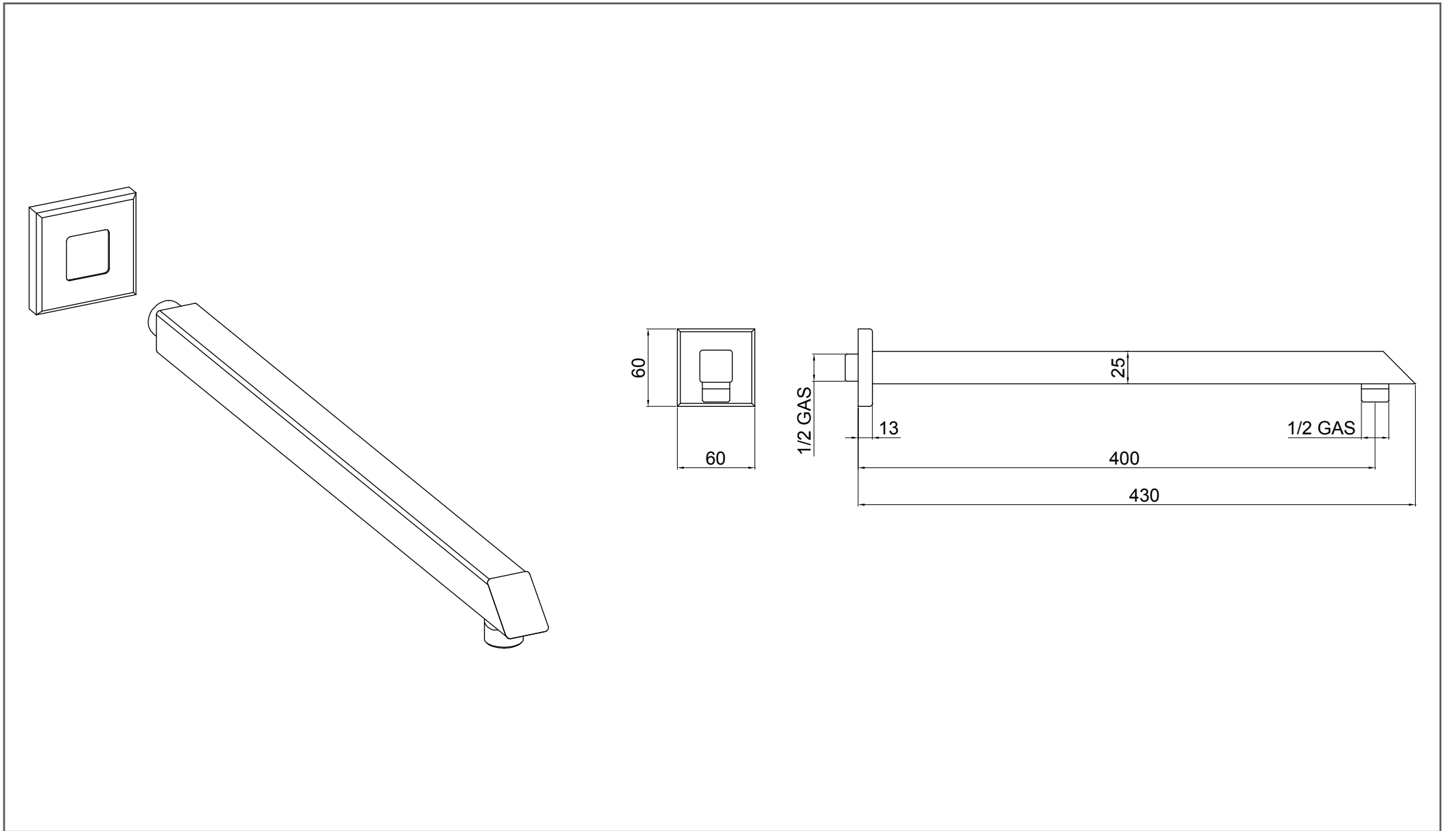
braccio quadro a muro wall arm square
